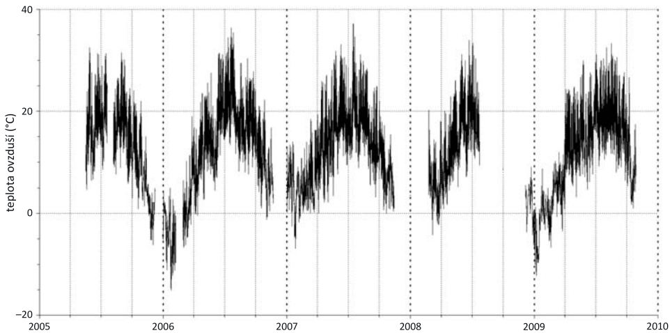
Obr. 9 – Hodinový vývoj teplot na meteorologické stanici Jezeří.
