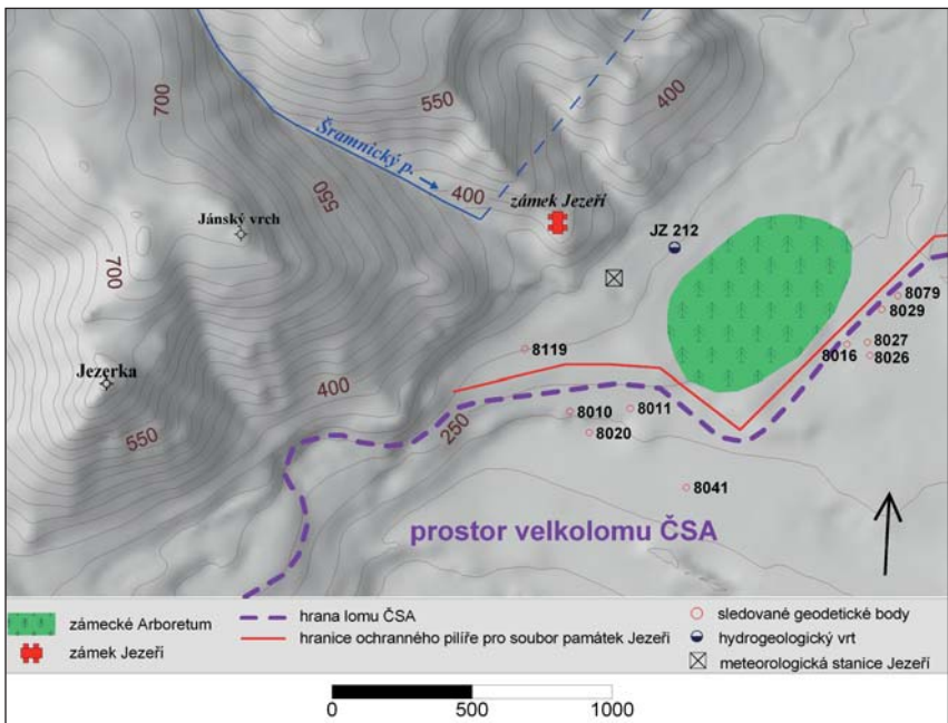
Obr. 5 – Přehledová mapa znázorňující lokalizaci deseti sledovaných geodetických bodů v prostoru stabilizačního pilíře pod zámekem Jezeří.
