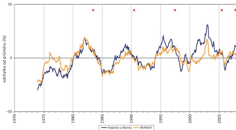
Obr. 6 – Odchylka od dlouhodobých měsíčních průměru srážek shlazená 36měsíčním klouzačným průměrem, značky představují vznik hluboce založeného sesuvu ve sledované lokalitě.
